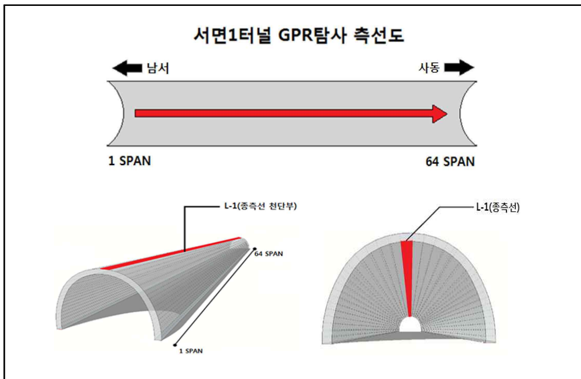
【그림 4.1-1】 축선위치도
