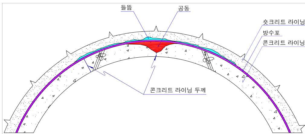
【그림 4.2-1】 콘크리트 라이닝 경계면 탐사모식도
